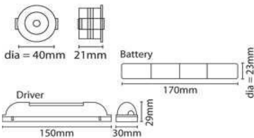
EPACK/LED2 & EPACK/LED3
